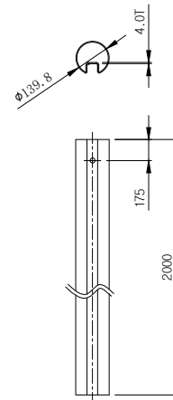
흙지주 SCALE: NONE
