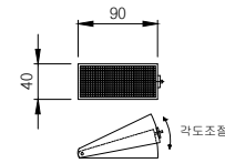
KD반사체 SCALE: NONE
