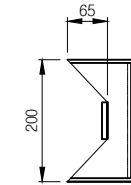
측면도
