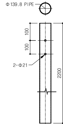
PIPE POST 상세도
