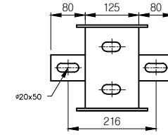
정면도
