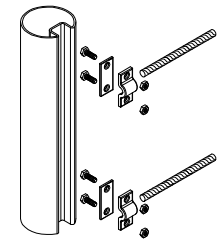
와이어고정구 사시도 SCALE: NONE
