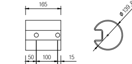
단부레일 SCALE: NONE
