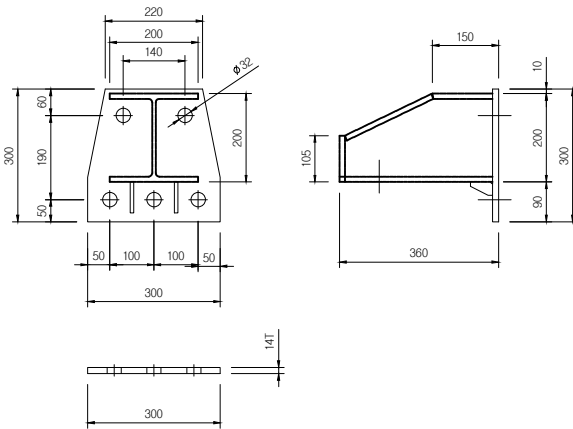
BASE PLATE SCALE: NONE
