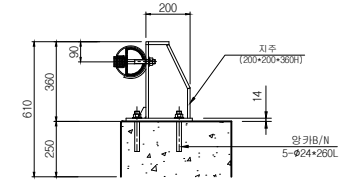
SIDE ELEVATION SCALE: NONE
