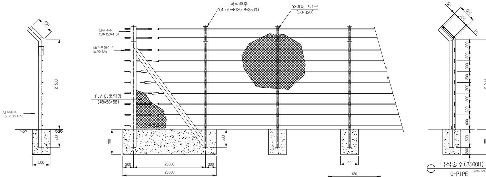
측면도 (단부지주)
