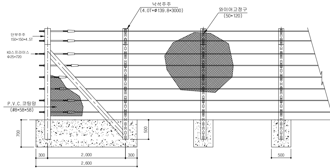
정면도
