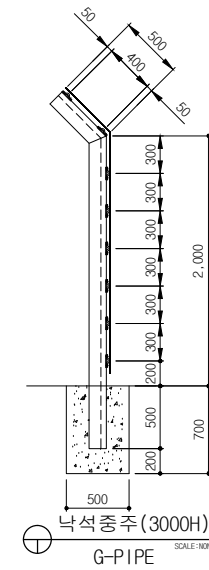
측면도 (중간지주)
