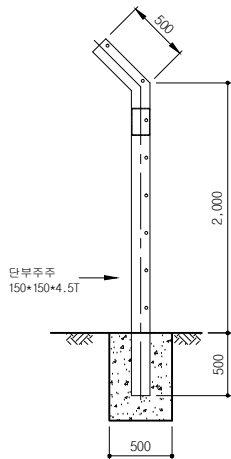
측면도 (단부지주)
